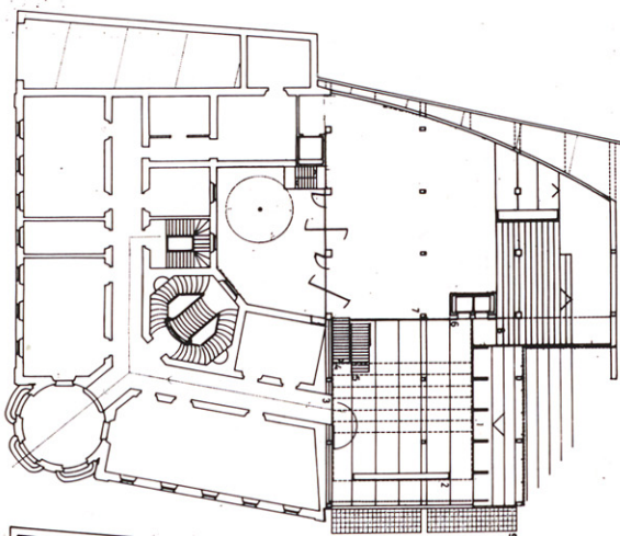
Planta (+ 1.10). Hall / 1. Entrada / 2. Mostrador información / 3. Conexión edificio existente / 4. Escalera a salas exposiciones / 5. Escalera a servicio público administrativo / 6. Ascensores / 7. Vacio sala exposiciones-actos / 8. Vacio entrada sala exposiciones-actos / 9. Lucernarios sala actos.
