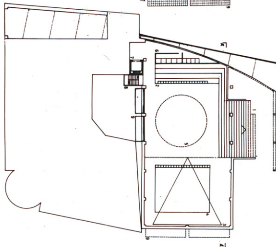
Planta (- 5.30). Sala de actos / 1. Escaleras de acceso / 2. Gradass / 3. Pantalla / 4. Butacas / 5. Posible escenario / 6. Aseos / 7. Ascensor / 8. Escalera incendios / 9. Lucernarios.
