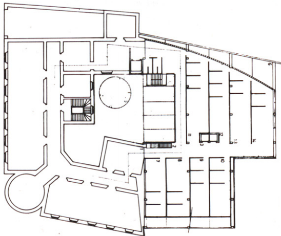
Planta (+ 680). Gobierno Gestión política / 1. Entrada por edificio existente / 2. Salón de plenos / 3. Sala de permanentes / 4. Sala de reuniones / 5. Sala prensa / 6. Lucernario / 7. Ascensores / 8. Escalera incendios / 9. Aseos / 10. Vacio entrada sala exposiciones-actos / 11. Vacio hall / 12. Vacio rampa parking.
