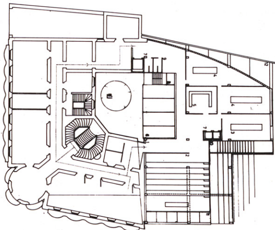
Planta (+ 680). Gobierno Gestión política / 1. Entrada por edificio existente / 2. Salón de plenos / 3. Sala de permanentes / 4. Sala de reuniones / 5. Sala prensa / 6. Lucernario / 7. Ascensores / 8. Escalera incendios / 9. Aseos / 10. Vacio entrada sala exposiciones-actos / 11. Vacio hall / 12. Vacio rampa parking.
